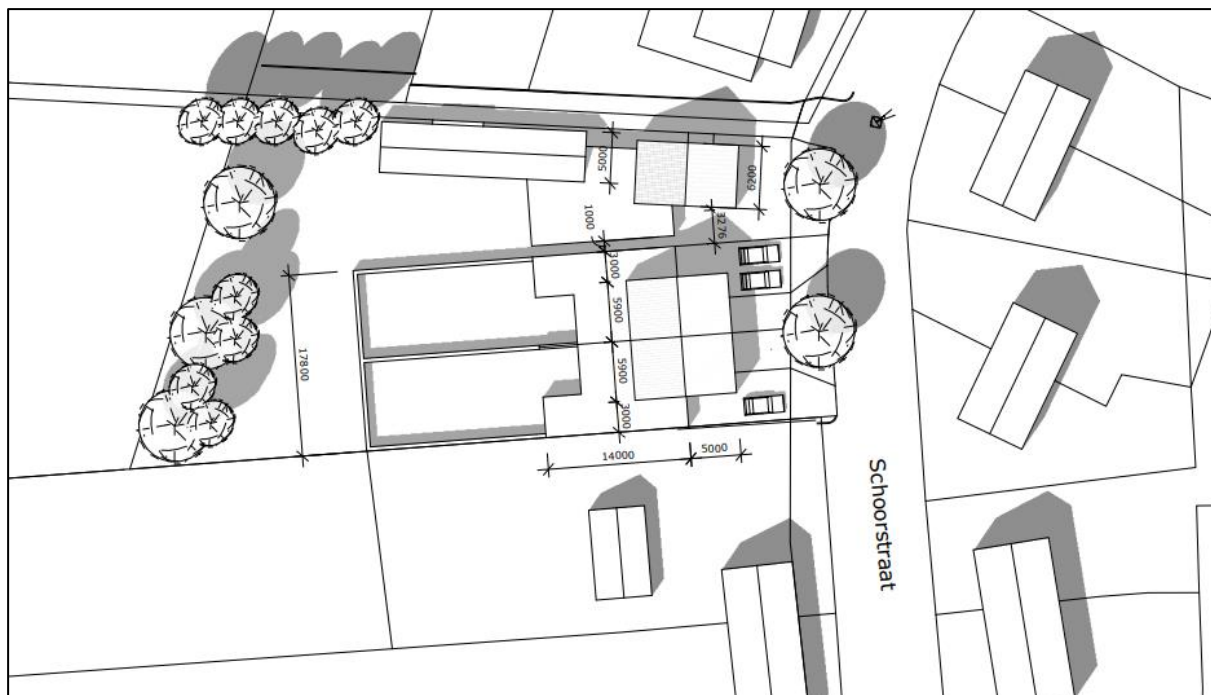
Figuur 13. Inrichtingsplan.
