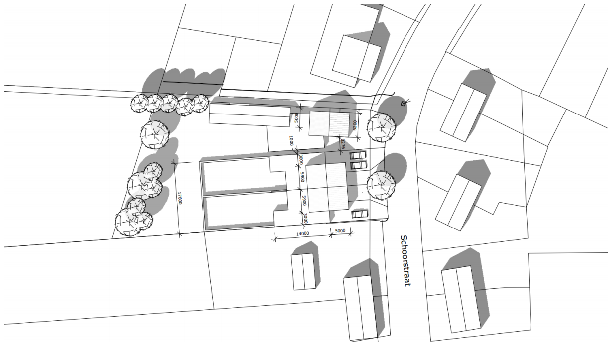
Figuur 2: Situatie tekening nieuwe situatie
