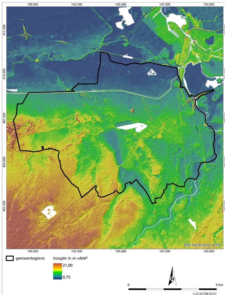
Afb. 7.1 Hoogtekaart (Afn-3) voor de gemeente Vught. De hoger gelegen gebieden zijn aangegeven in bruin-oranje-geel, de lager gelegen gebieden (beekdalen en Gement) zijn groen-blauw. Het witte vlak binnen de gemeentegrens is de zandafgraving IJzeren Man.
