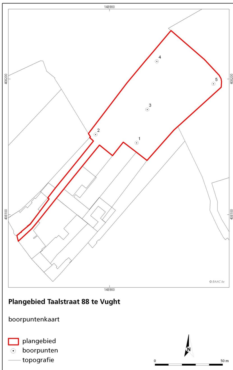
Figuur 3.1 Boorpuntenkaart
