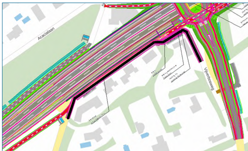
Afbeelding 3.18: Ontwerp parallelweg De Bréautelaan - Boslaan (zwarte lijn)
