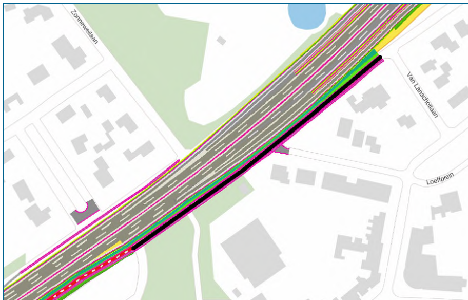
Afbeelding 3.14: Ontwerp parallelweg Helvoirtseweg (zwarte lijn)
