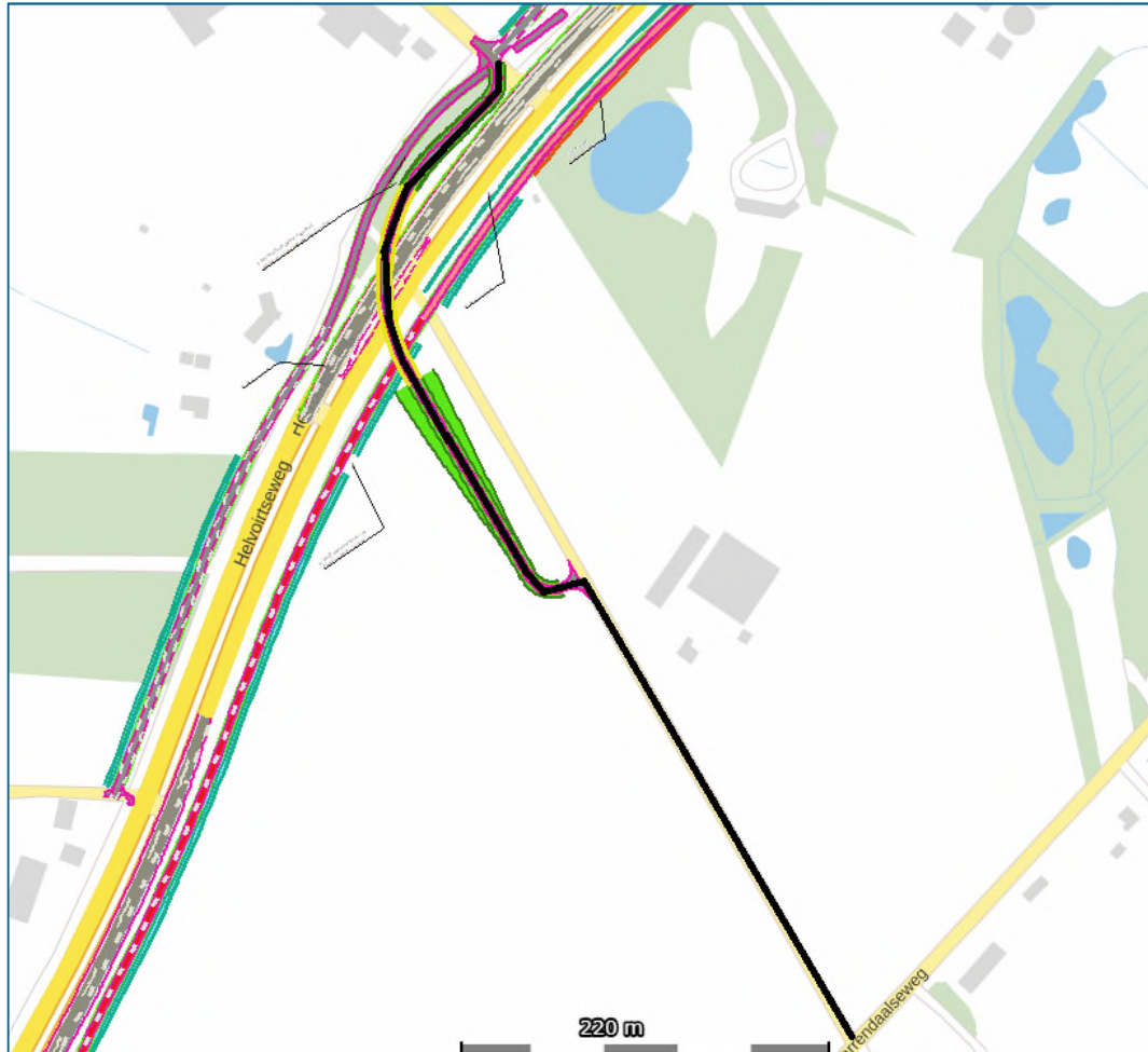
Afbeelding 3.9: Ontwerp nieuw viaduct Kruishoeveweg - Sparrendaalseweg
