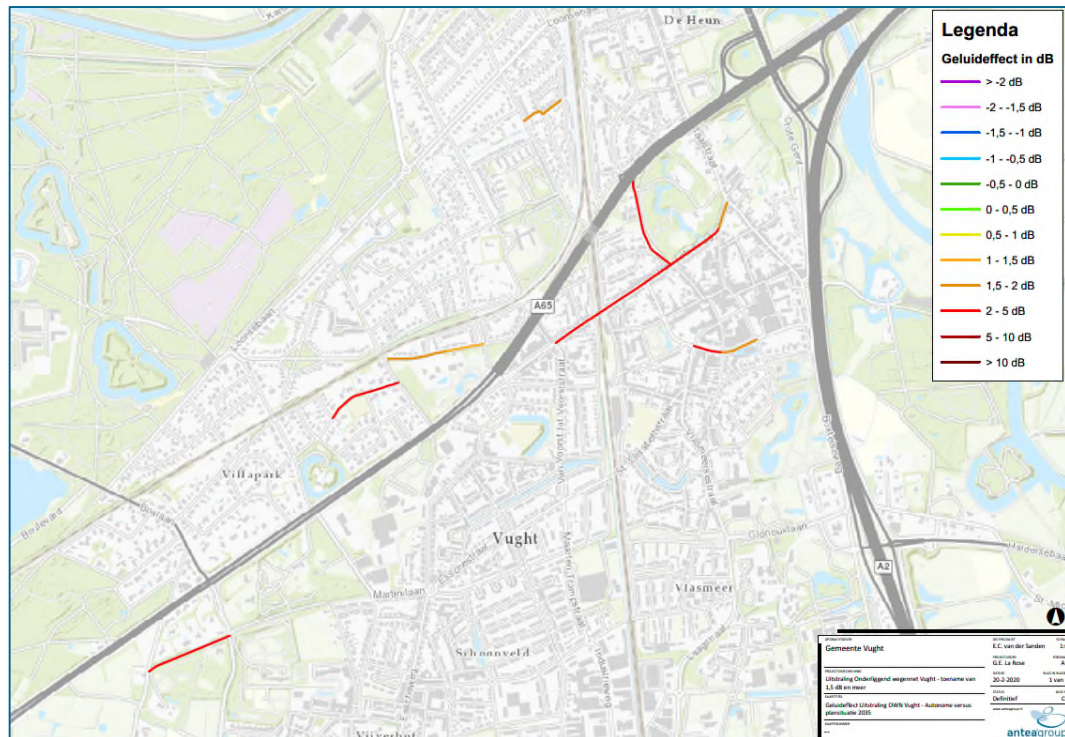
Afbeelding 6.3: Toenames geluidbelasting van 1,5 dB of meer, rekening houdend met selectiecriteria
