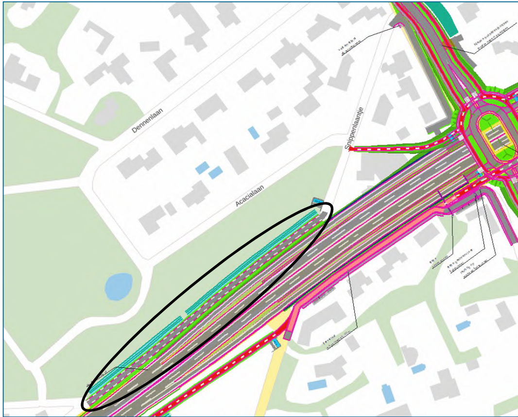
Afbeelding 3.17: Ontwerp parallelweg Snippenlaantje - Cromvoirtsepad (zwart omcirkeld)
