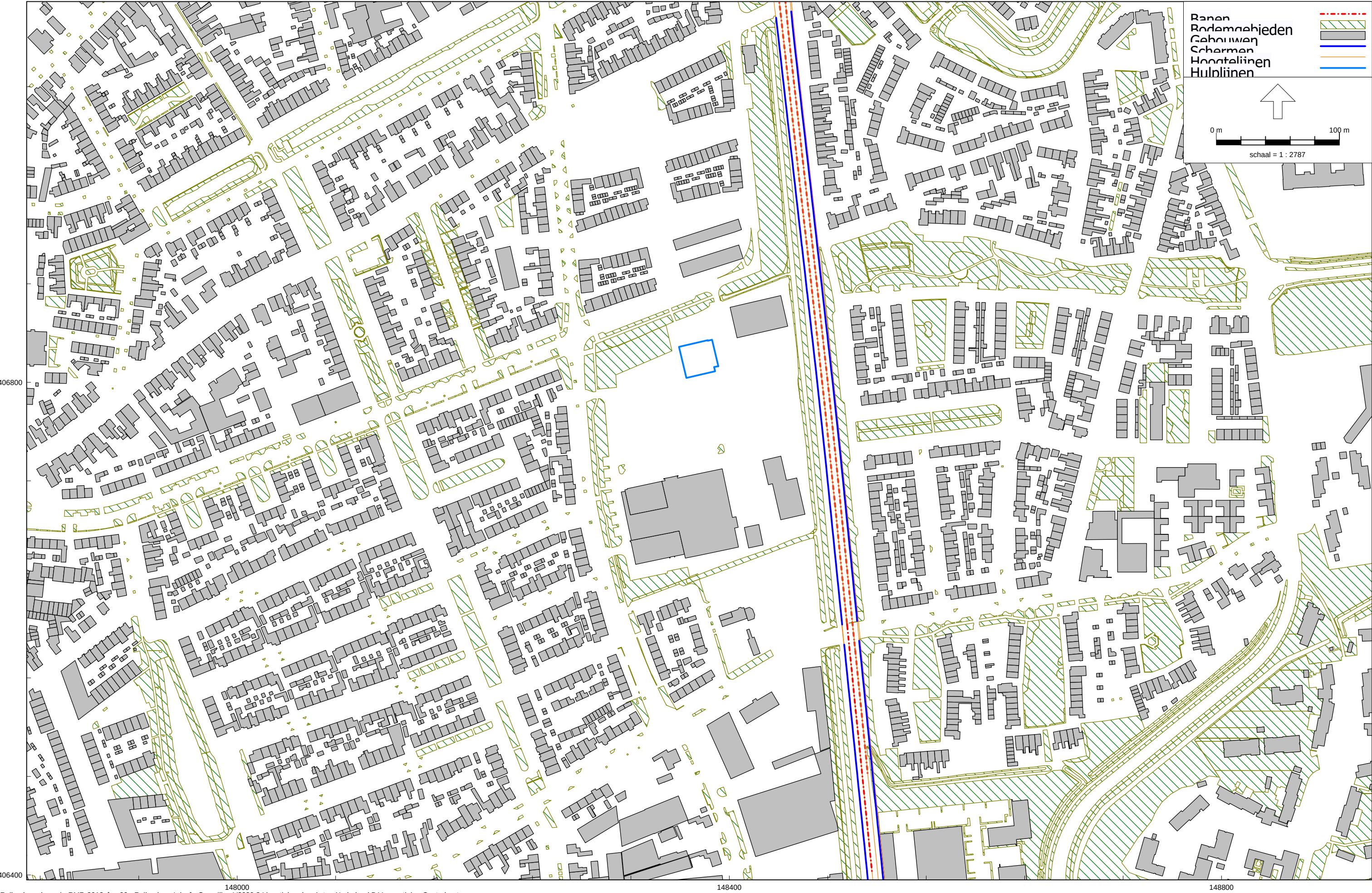
Overzicht rekenmodel railverkeerslawaa
