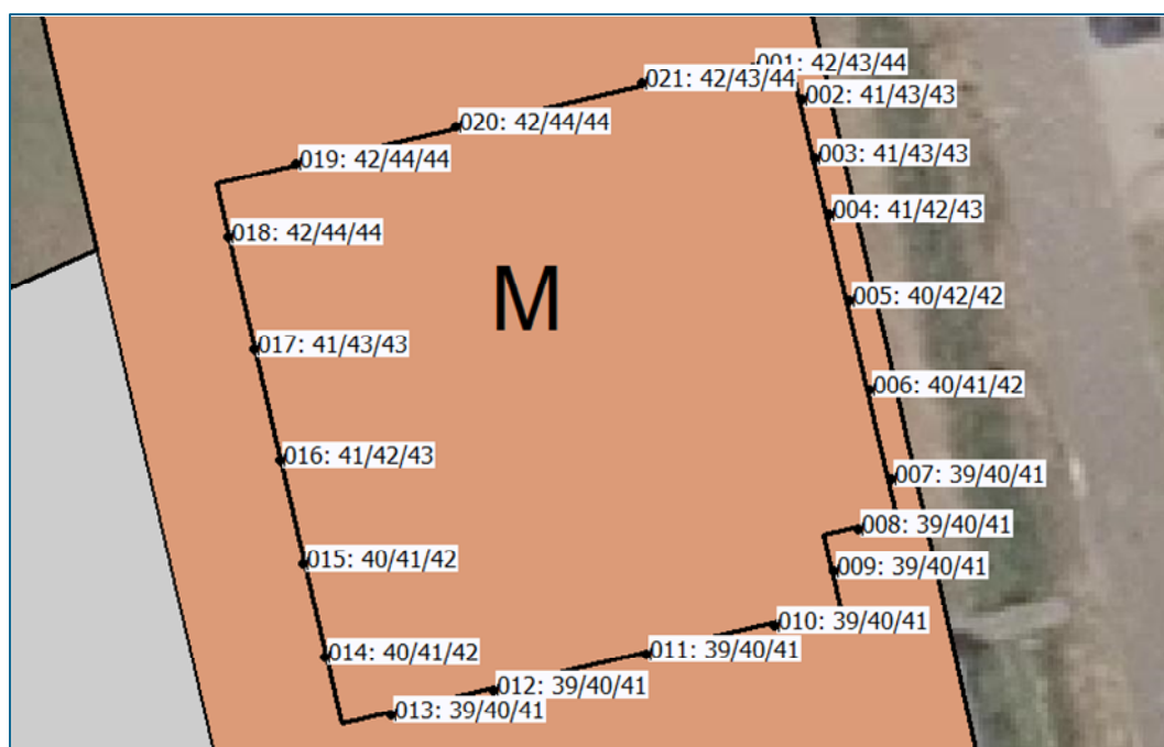
Afbeelding 4.1: Overzicht resultaten Michiel de Ruyterweg incl. aftrek [dB L dag ]
