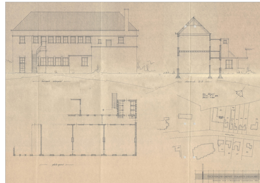
Boven: tekening 'bestaande situatie' in 1953 kort voor de ophoging met één bouwlaag. Onder: tekening 'bestaande situatie' in 1990 kort voor de uitbreiding aan de achterzijde (bron: BHIC bouwdoSSIERS gemeente Vught) .
