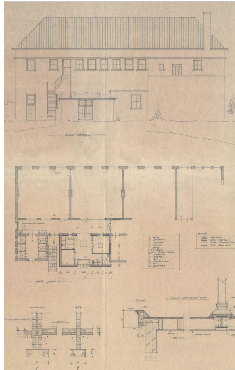
Links: tekening 'nieuwe situatie' in 1990 met de uitbreiding van de peuterzaal op de begane grond. Rechts: uitsnede tekening 'bestaande en nieuwe situatie' uit 1972 van de begane grond van de schoolmeesterswoning (bron: BHIC bouwdoSSIERS gemeente Vught).
