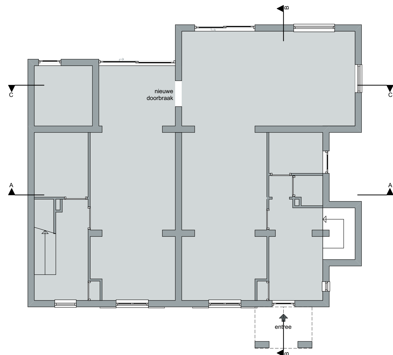
Begane grond
