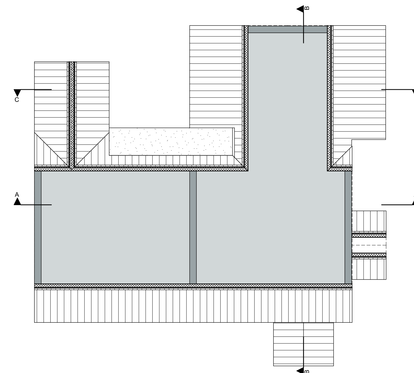
2e verdieping
