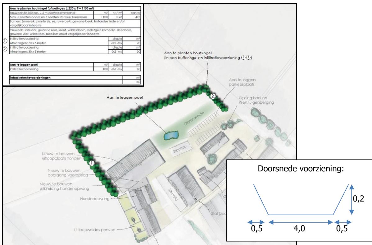
Abbeelding 17: weergave beoogde infiltratiesloot met doorsnede-tekening
