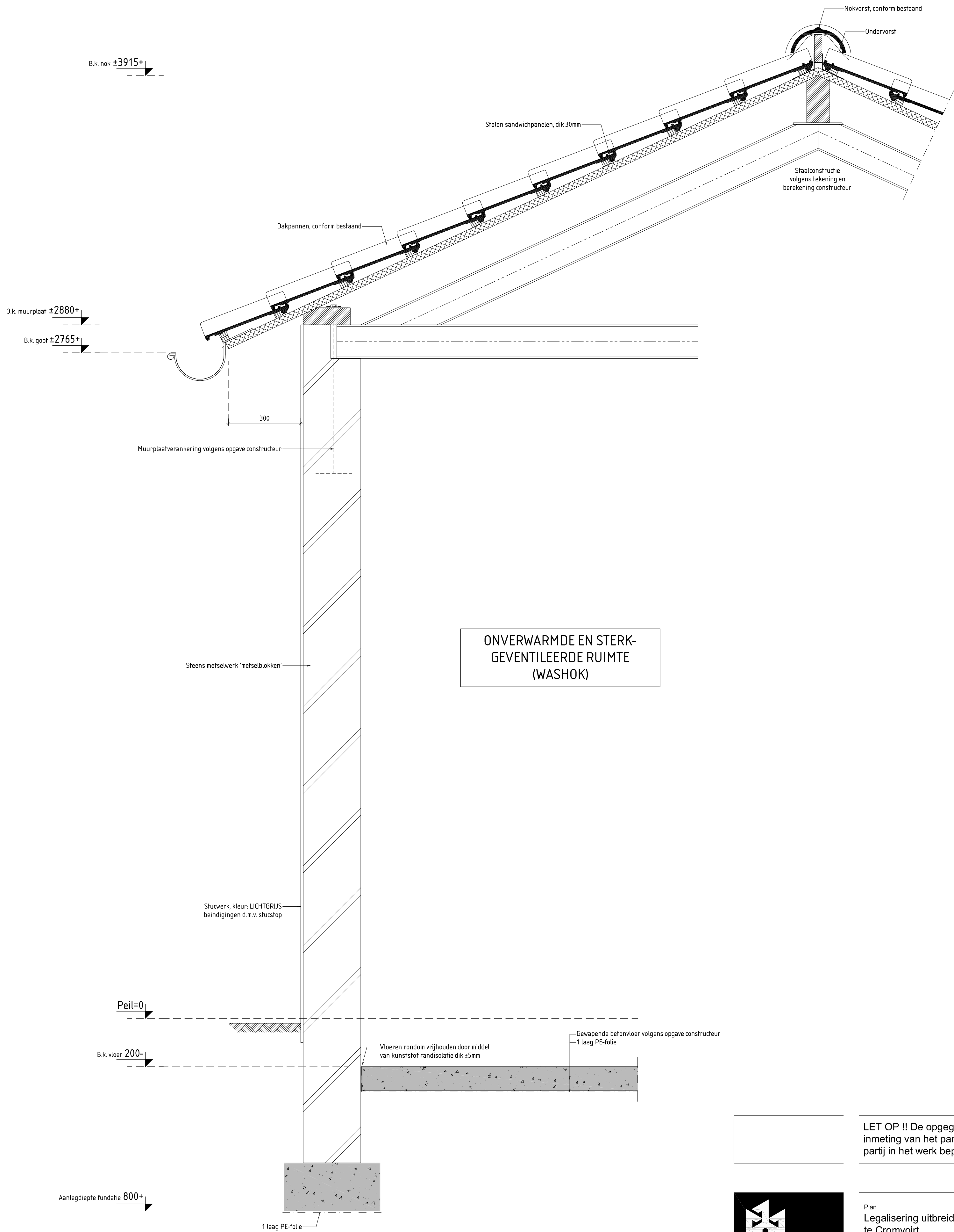
PRINCIPEDETAIL t.p.v. WASHOK (linker zijgevel)
