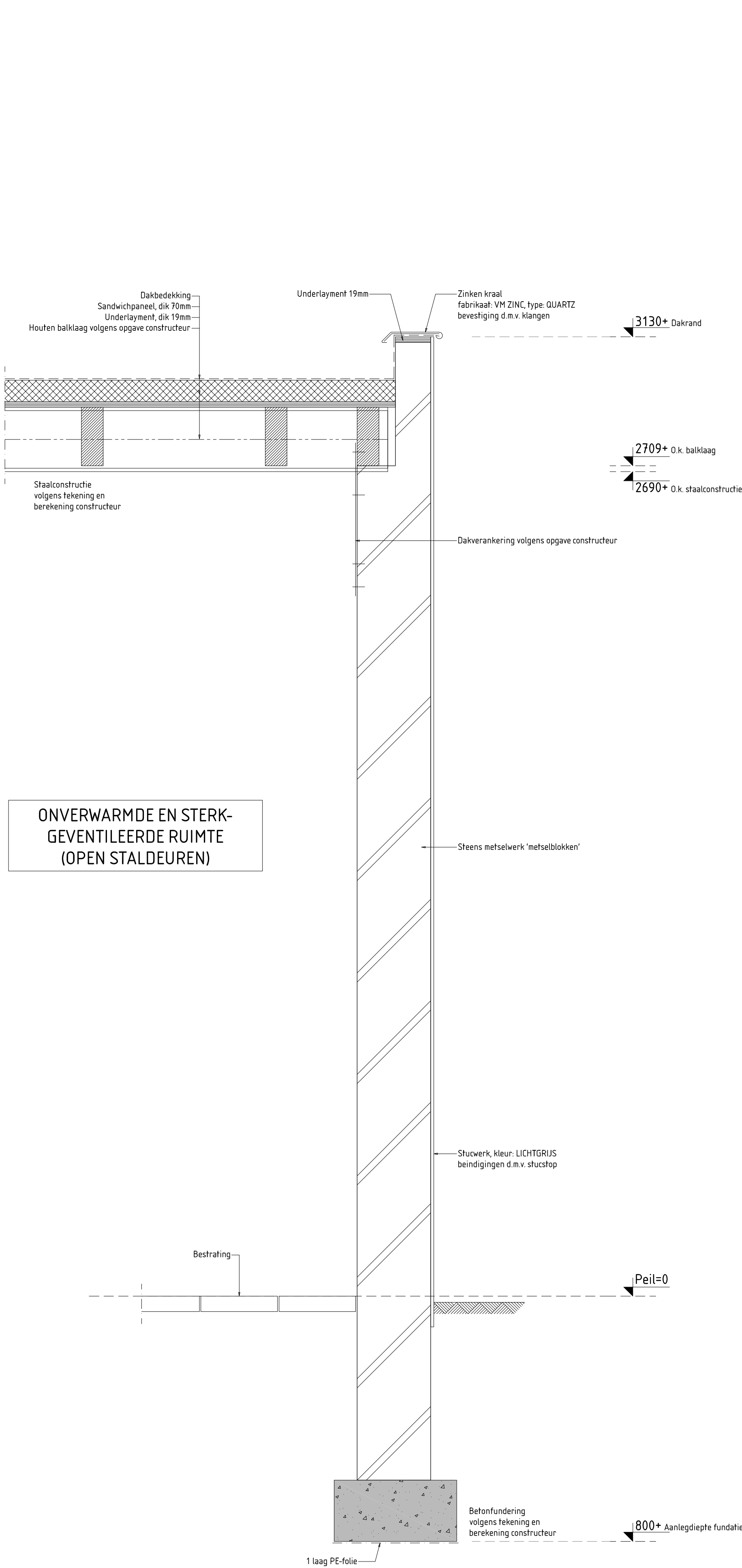
PRINCIPEDETAIL t.p.v. STALLEN (voorgevel)
