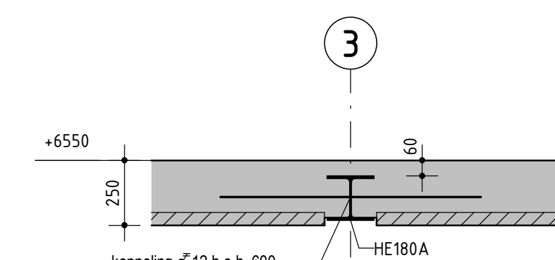
DSN. 2.01
