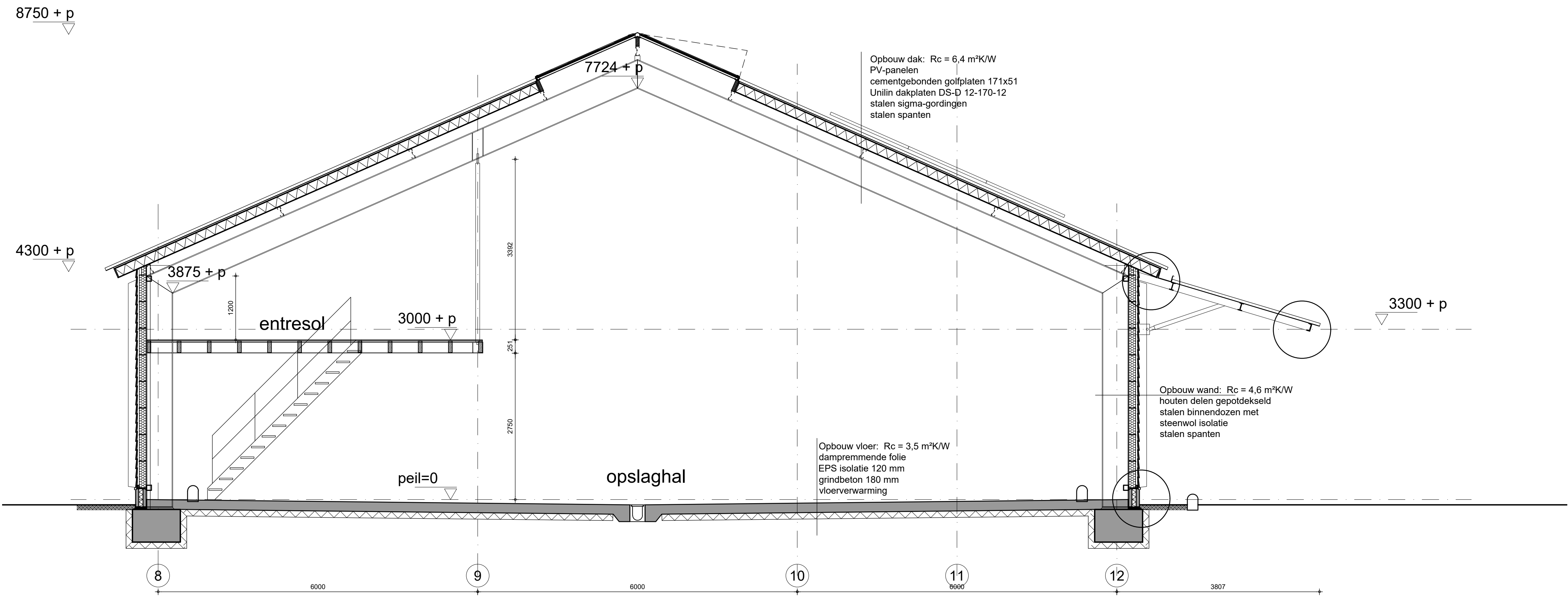
doorsnede CC
