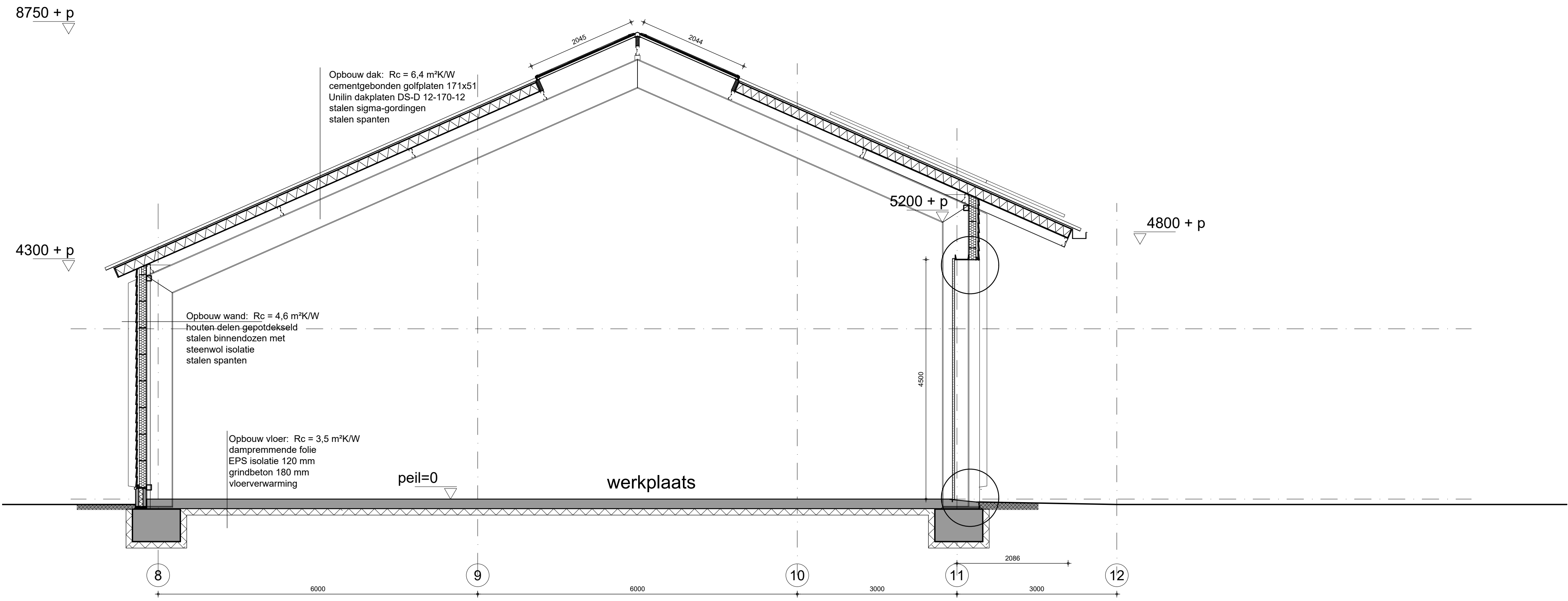
doorsnede DD
