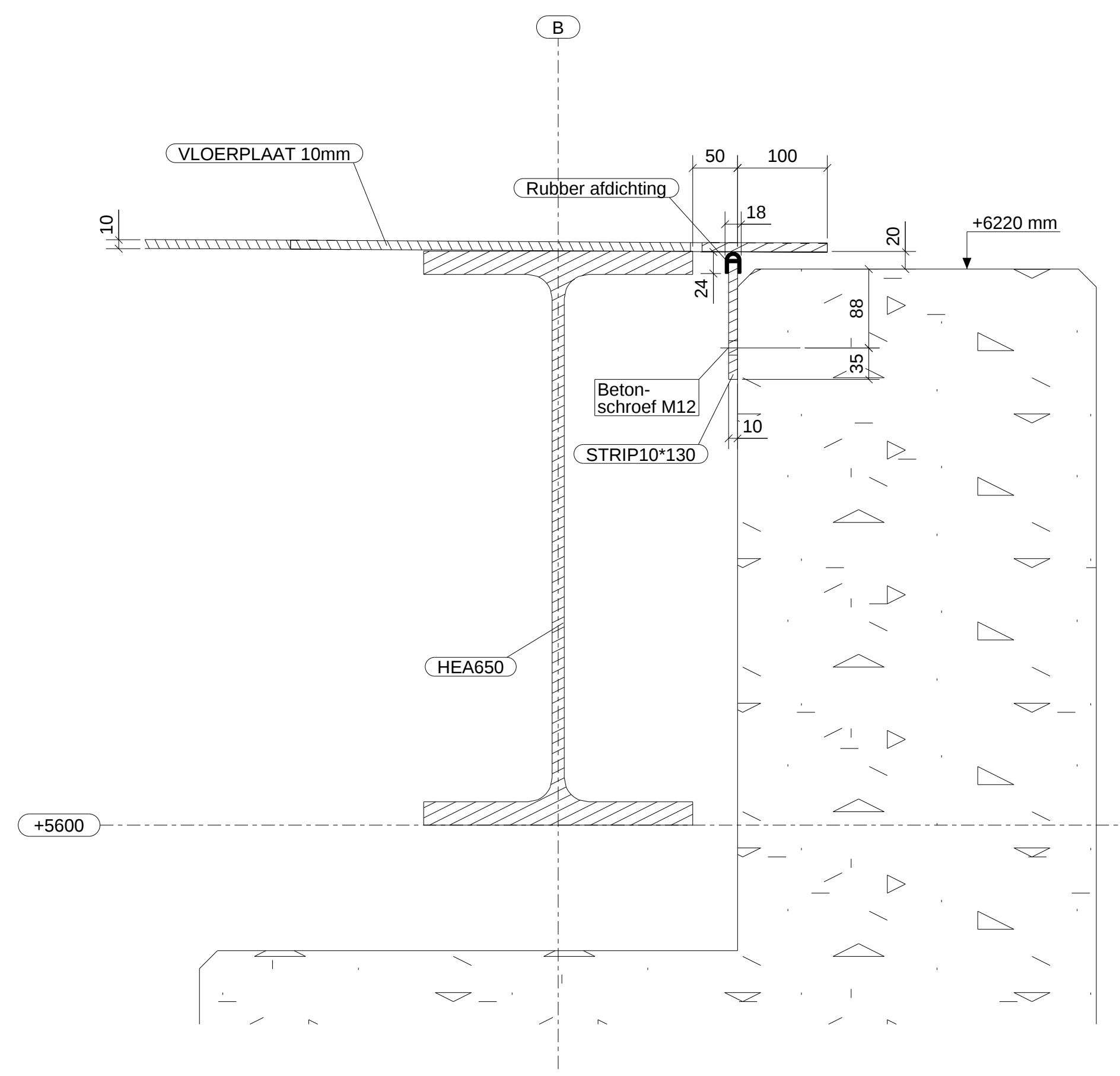
DETAIL VLOERRAND T.H.V. VOEGOVERGANG PLANTENBAK 1:5
