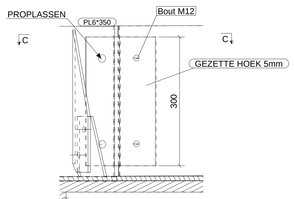
TYP. DETAIL KOPPELING VLOERRAND T.H.V. VOEGOVERGANG 1:5
