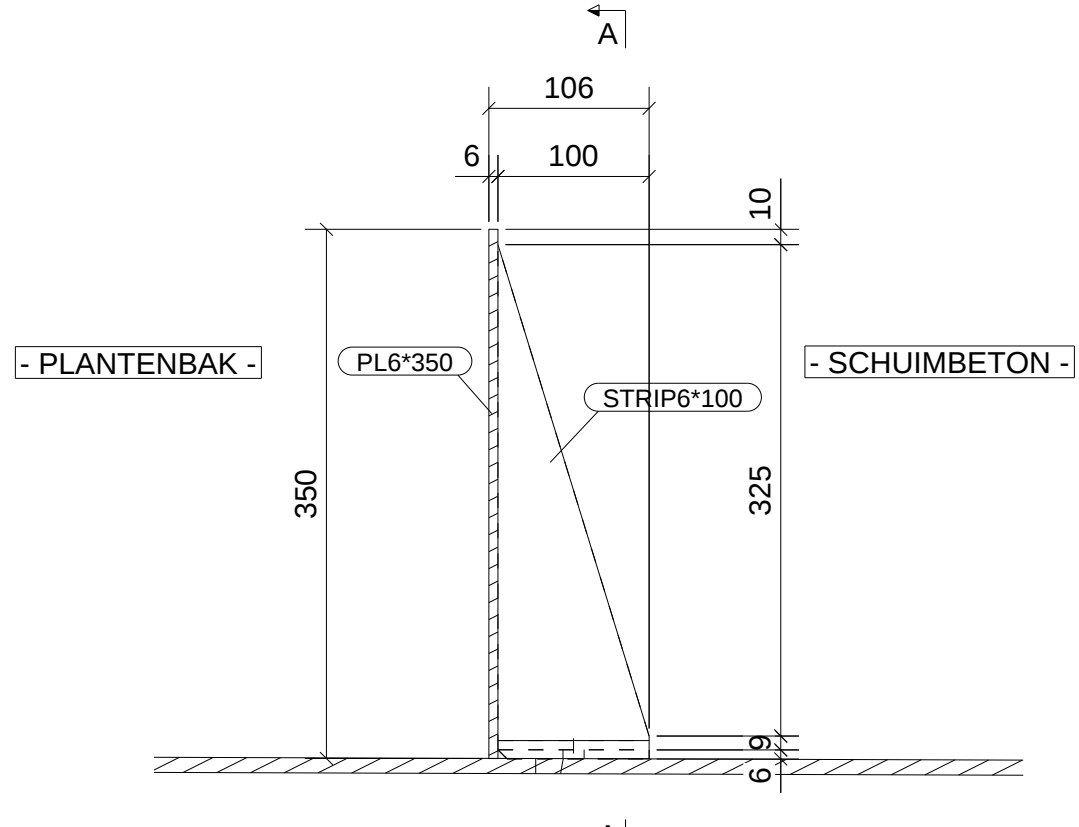
TYP. DETAIL VLOERRAND 1:5
