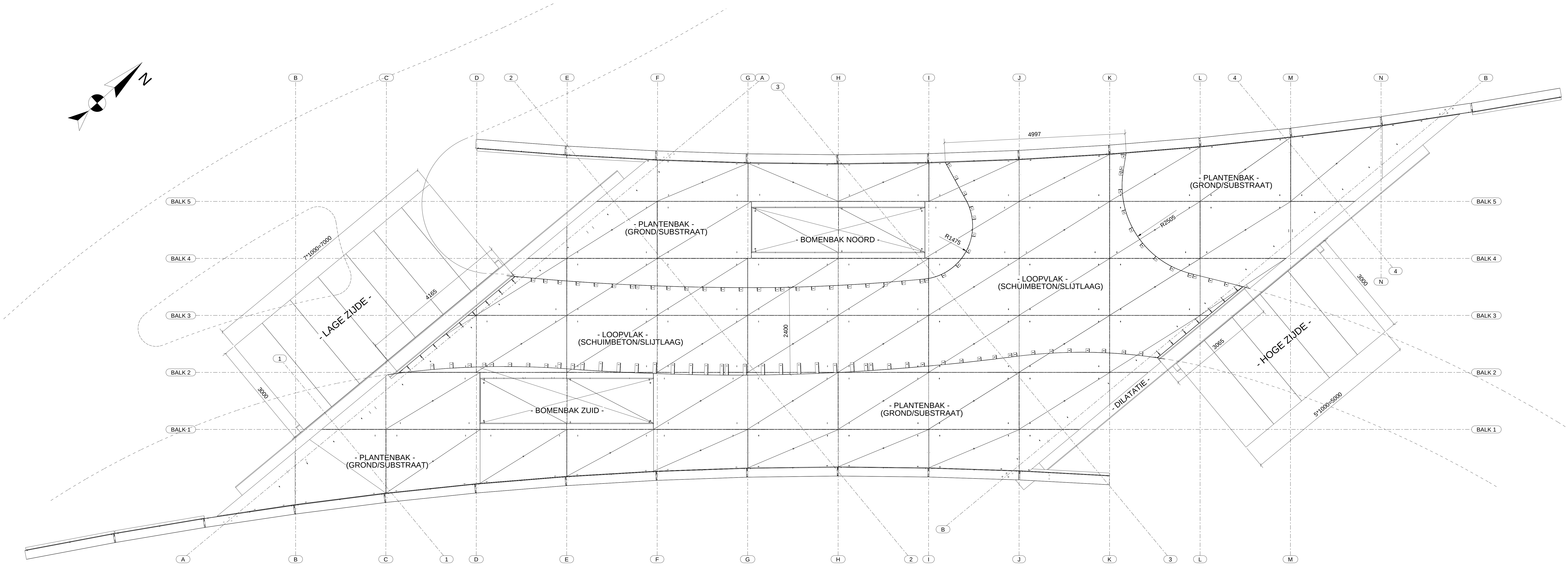
BOVENAANZICHT BRUGDEK 1:40
