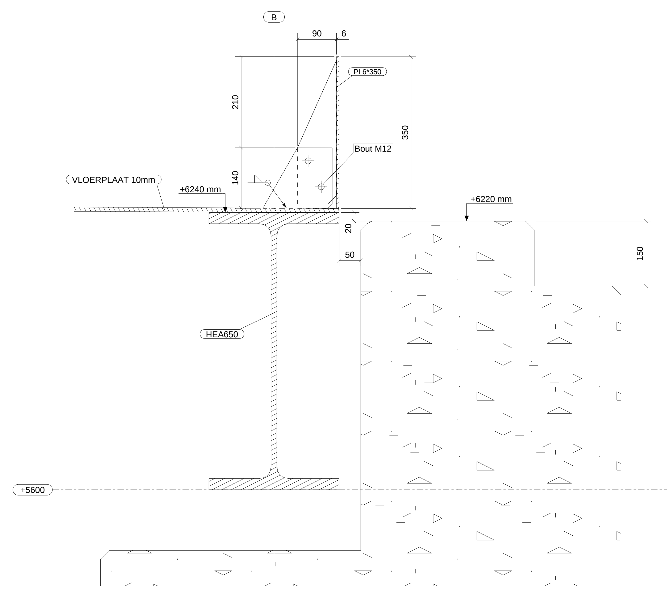
DETAIL VLOERRAND T.H.V. VOEGOVERGANG LOOPPAD 1:5
