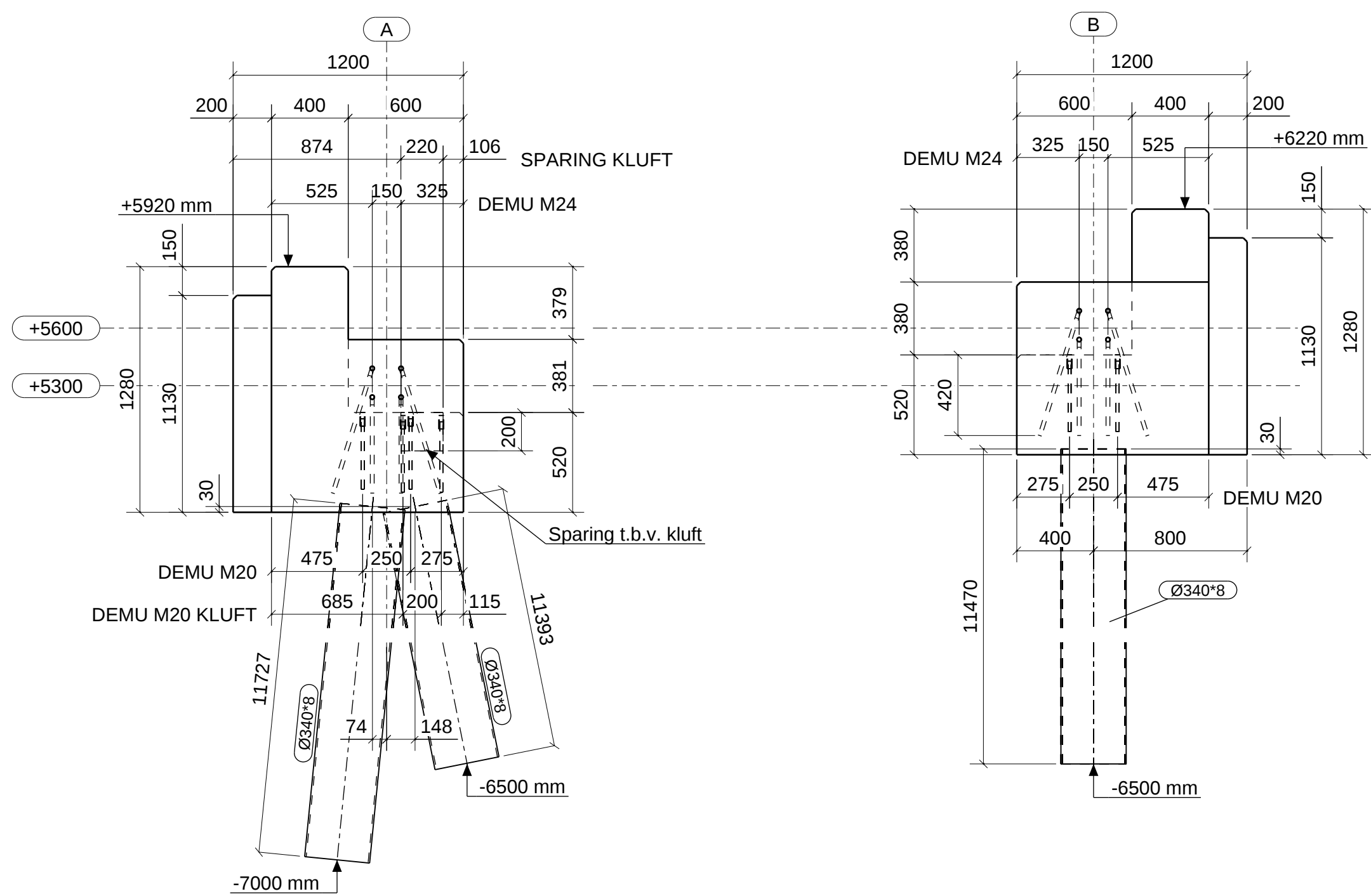
Haaks aanzicht 1:25
