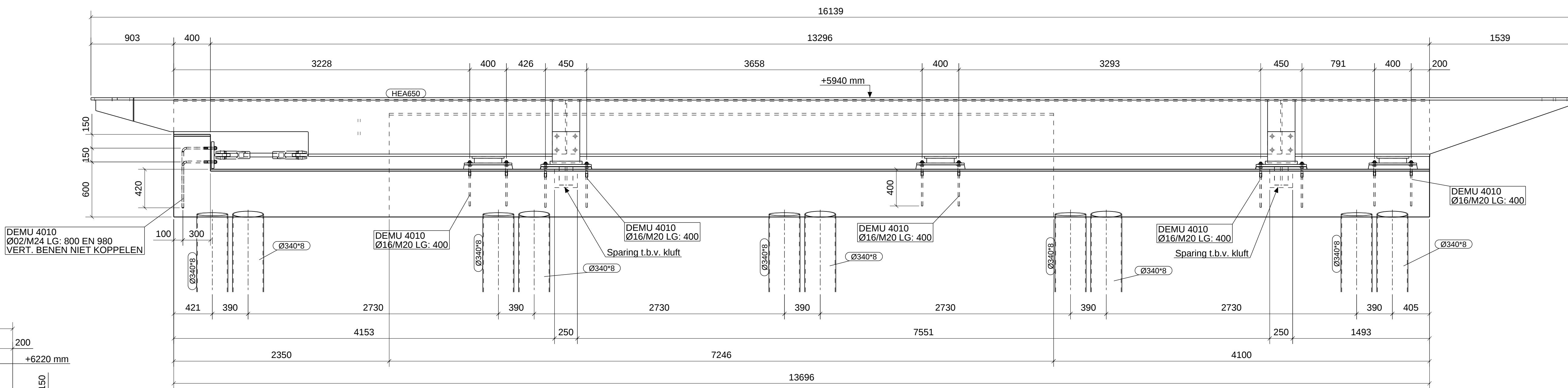
Doorsnede A - A 1:25
