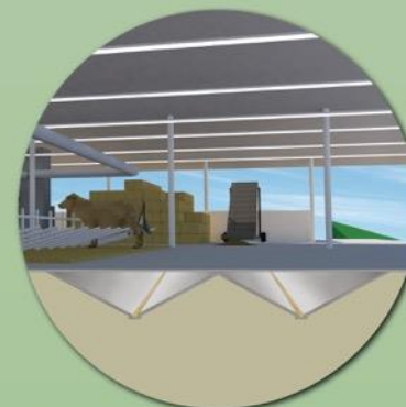
Vloer met gescheiden opvang vaste (stro)mest en vloeibare mest
