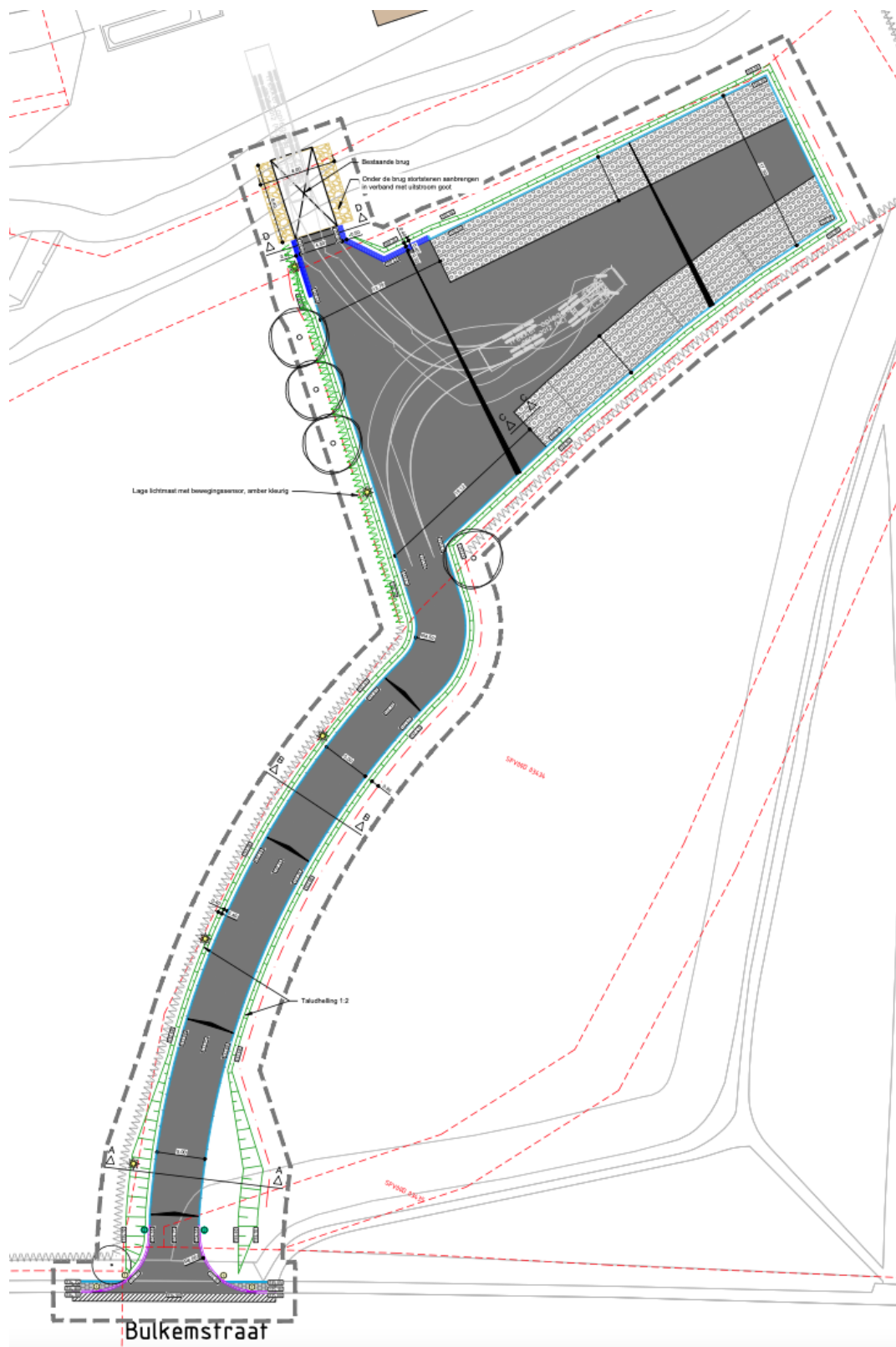
Afbeelding 7: Situatietekening toegangsweg en parkeerterrein
