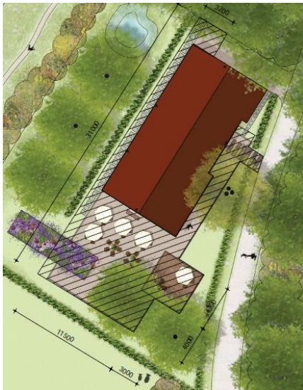
Situatietekening
