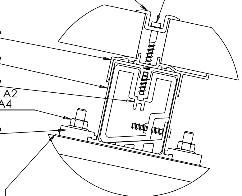
DETAIL F VERHOUDING 1:2
