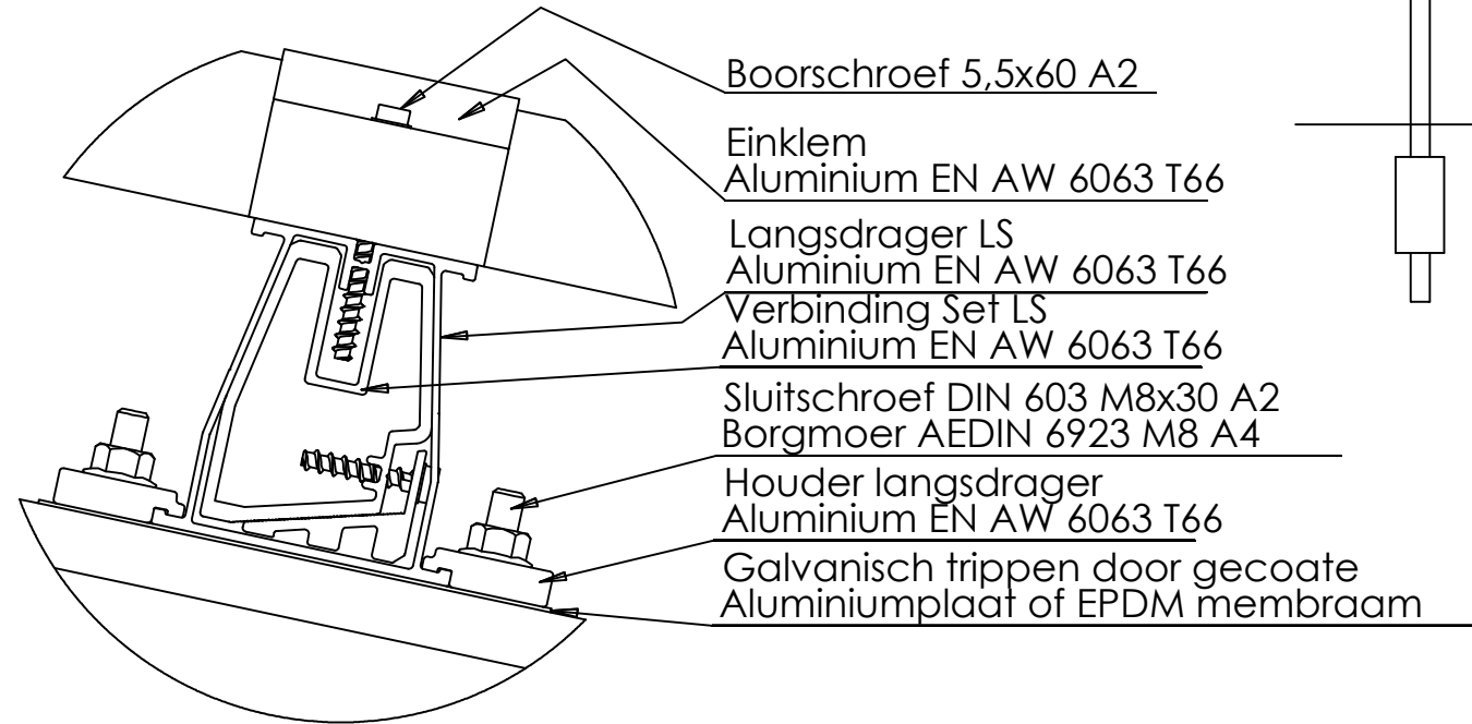
DETAIL E VERHOUDING 1:2
